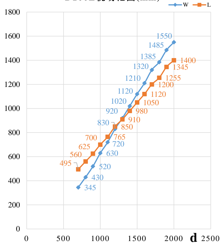
D100L视场范围(mm)
