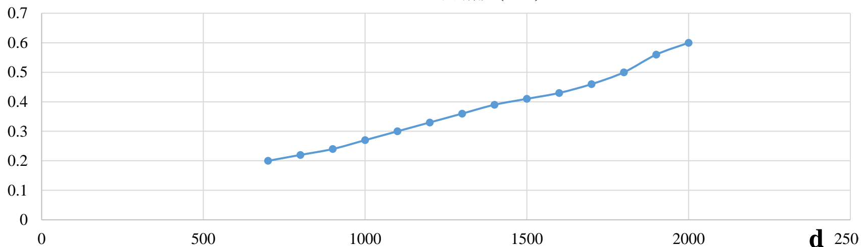
D100L点云Z向精度(mm)
